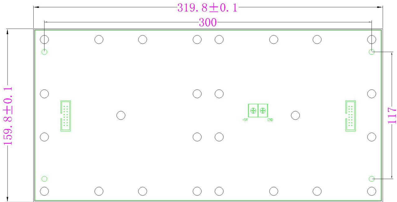
底视图
